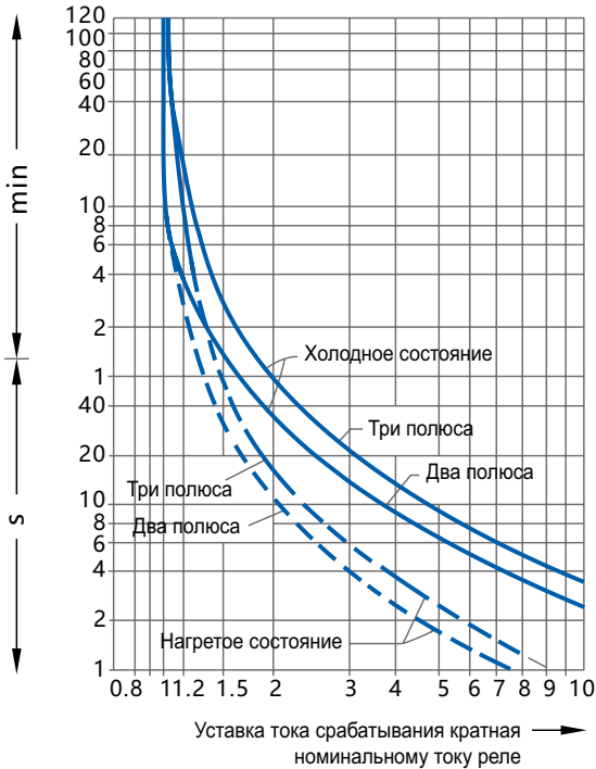
Время-токовая характеристика теплового реле (+20°)
